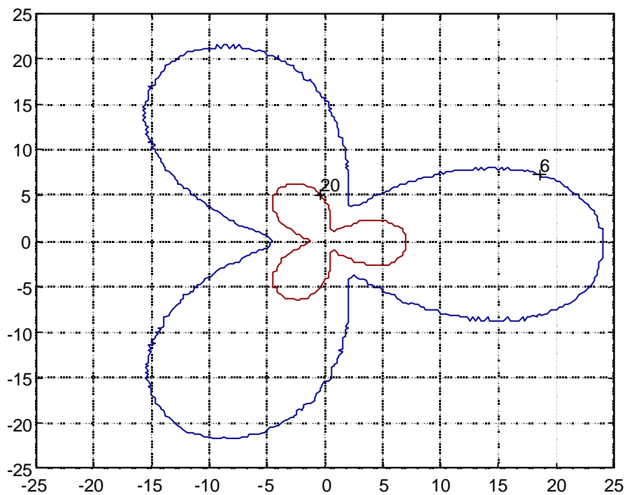
Figura 9 : esempio di zone di rispetto a 6 e 20 V/m
